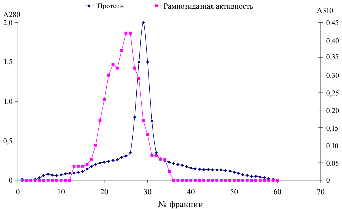
Рис. 5. Профиль элюции на TSK HW-60 препарата α-L-рамнозидазы C. albidus 1001
